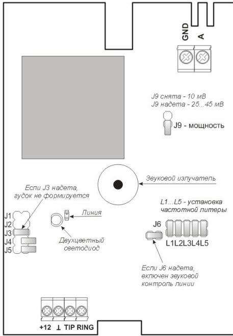
Рис. 2б. Монтажная схема RS-202TC-RR
