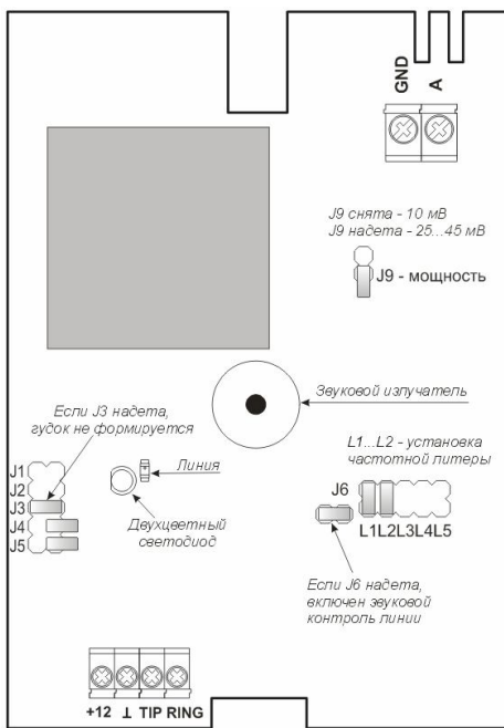
Рис. 2а. Монтажная схема RS-201TC-RR
