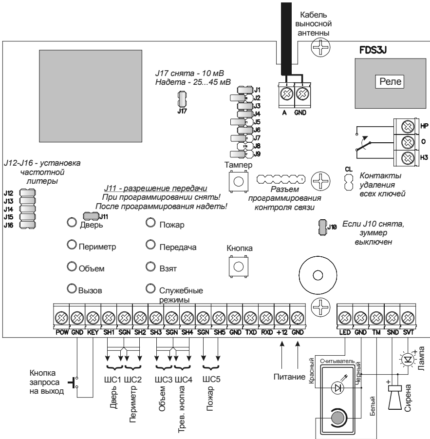
Рисунок 7 – Монтажная схема передатчика
