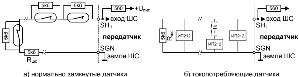
Рисунок 4 – Примеры монтажа пожарных шлейфов
