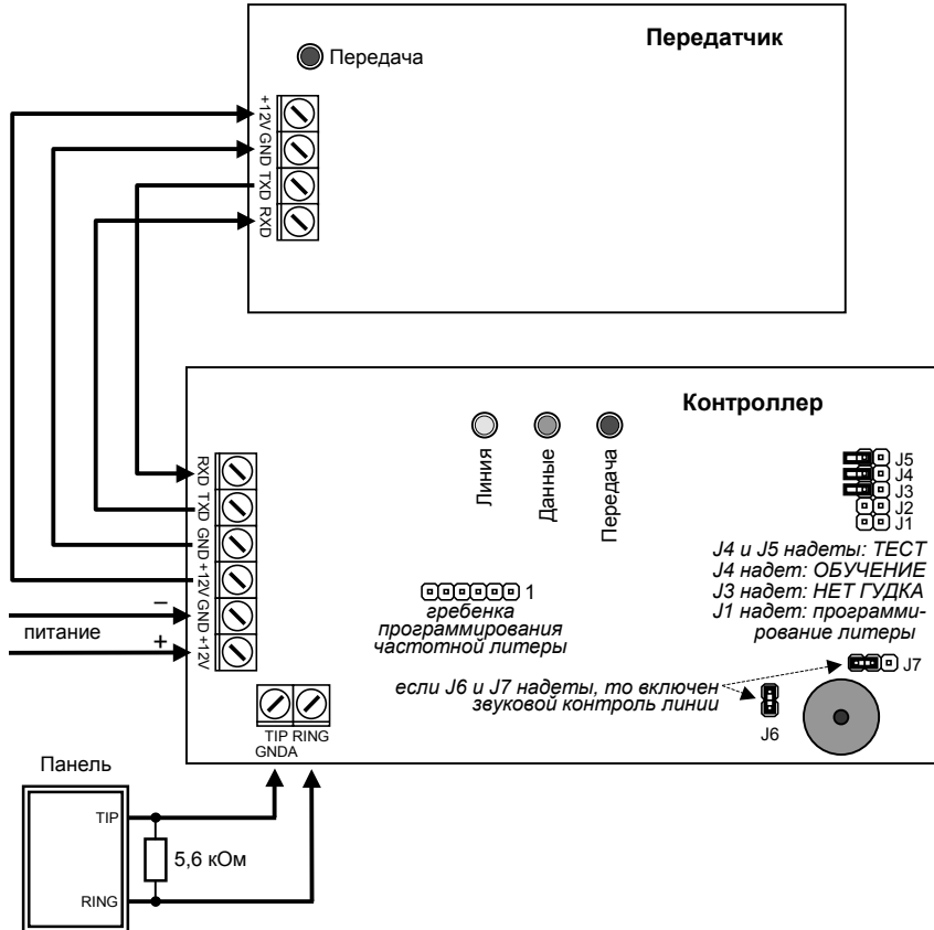
Рис. 2. Монтажная схема прибора
