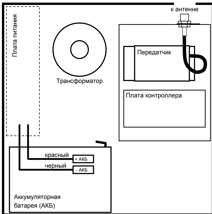
Рис. 1. Компоновка прибора
